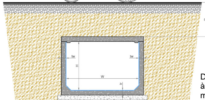
Plan de pose en t
