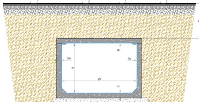
Plan de pose en b.a.
